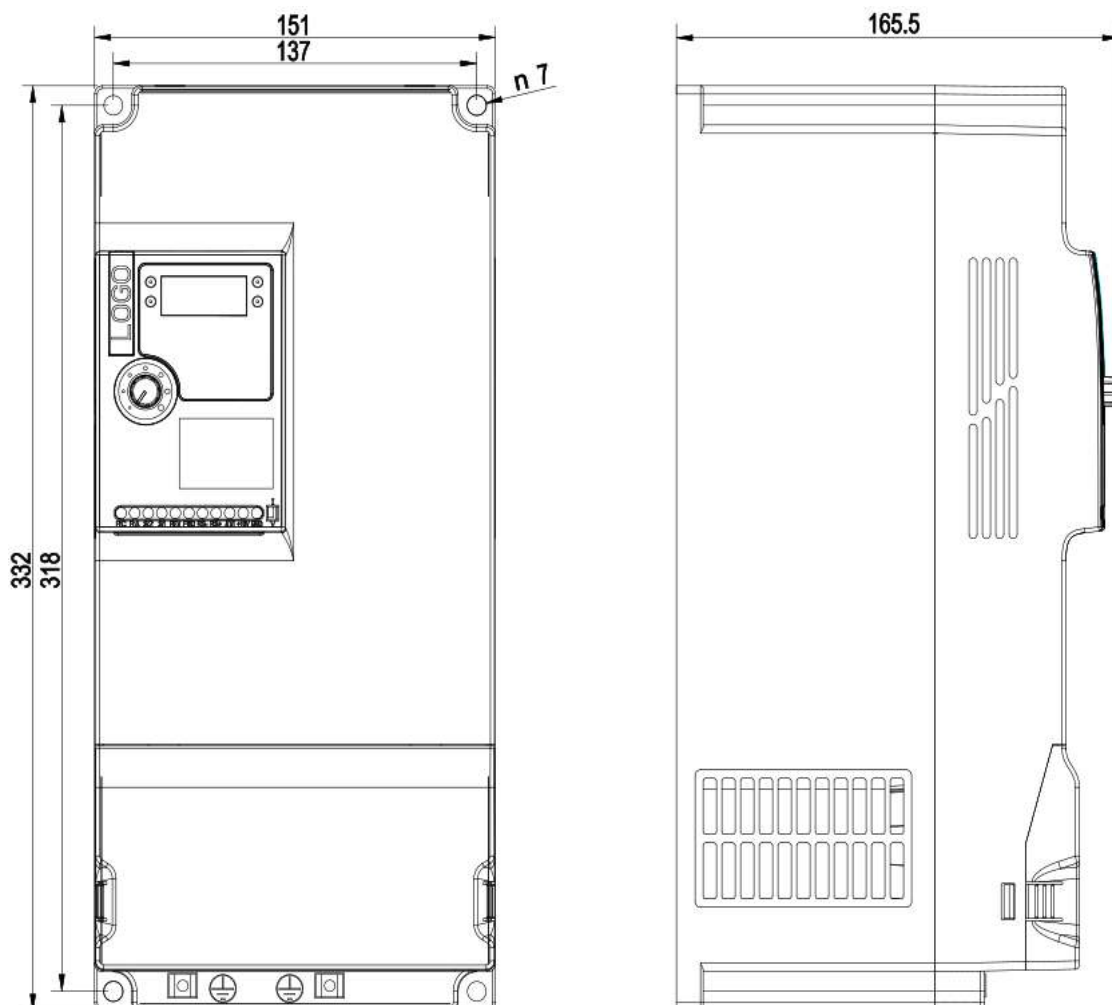
Rozmerový výkres A550 PLUS - 22kW 4T0220
