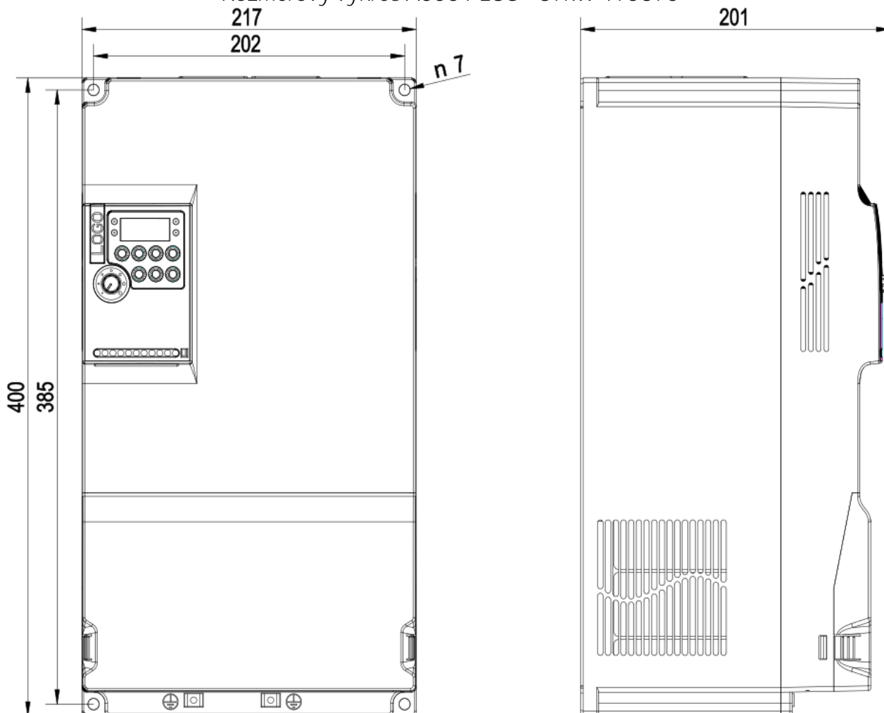
Rozmerový výkres A550 PLUS - 37kW 4T0370
