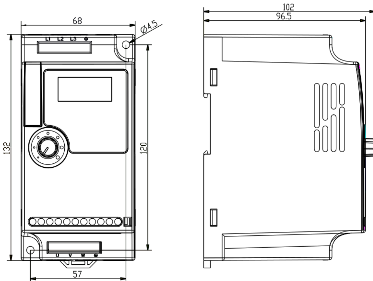
Rozmerový výkres A550 PLUS - 1,5kW 2S0015
