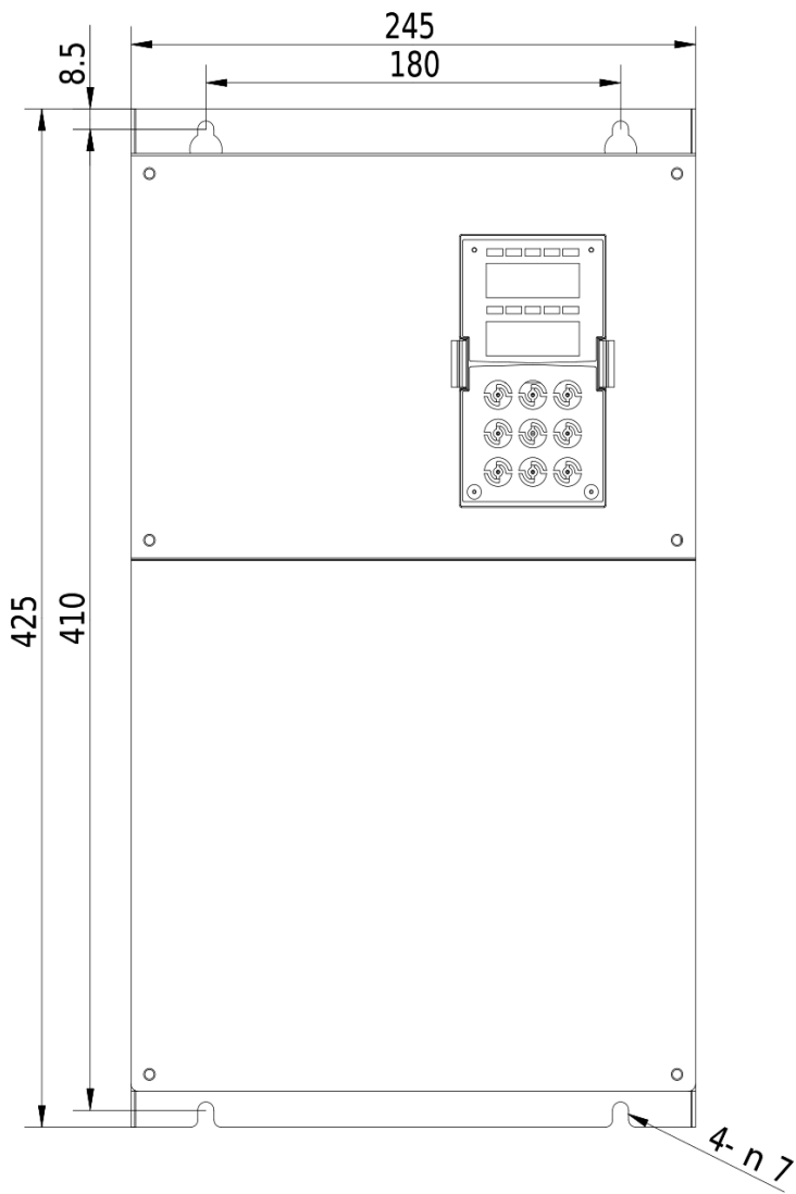
Rozmerový výkres V800 - 30kW 4T0300
