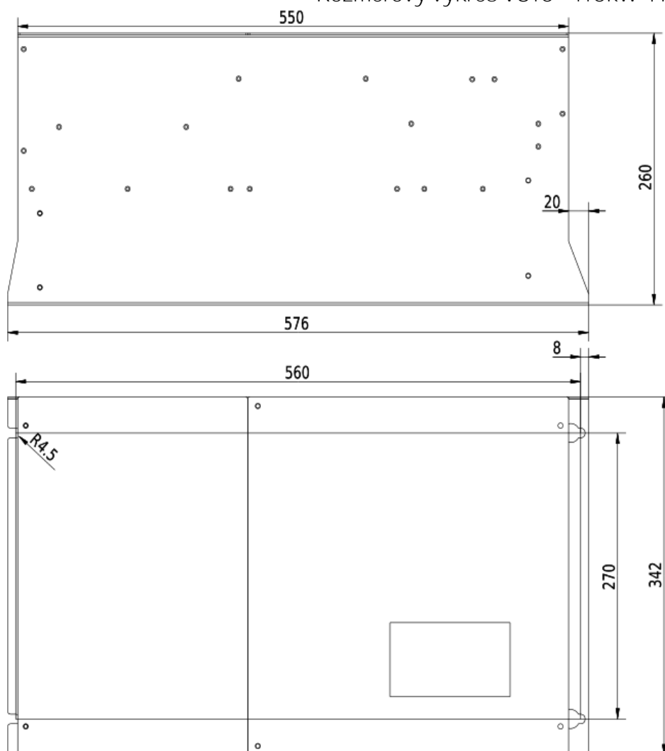
Rozmerový výkres V810 - 110kW 4T1100
