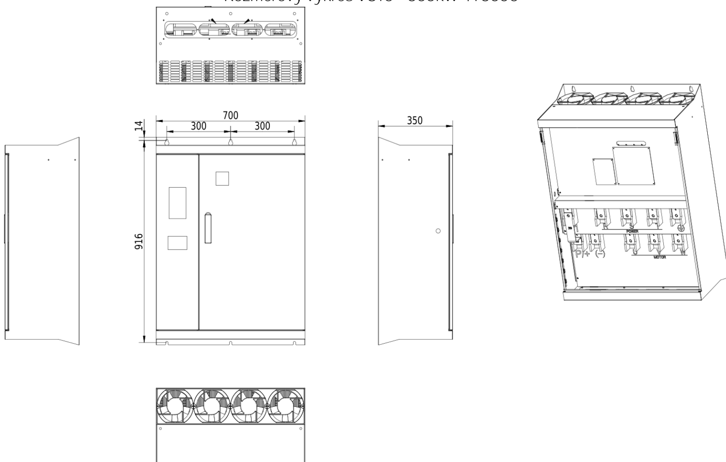
Rozmerový výkres V810 - 355kW 4T3550
