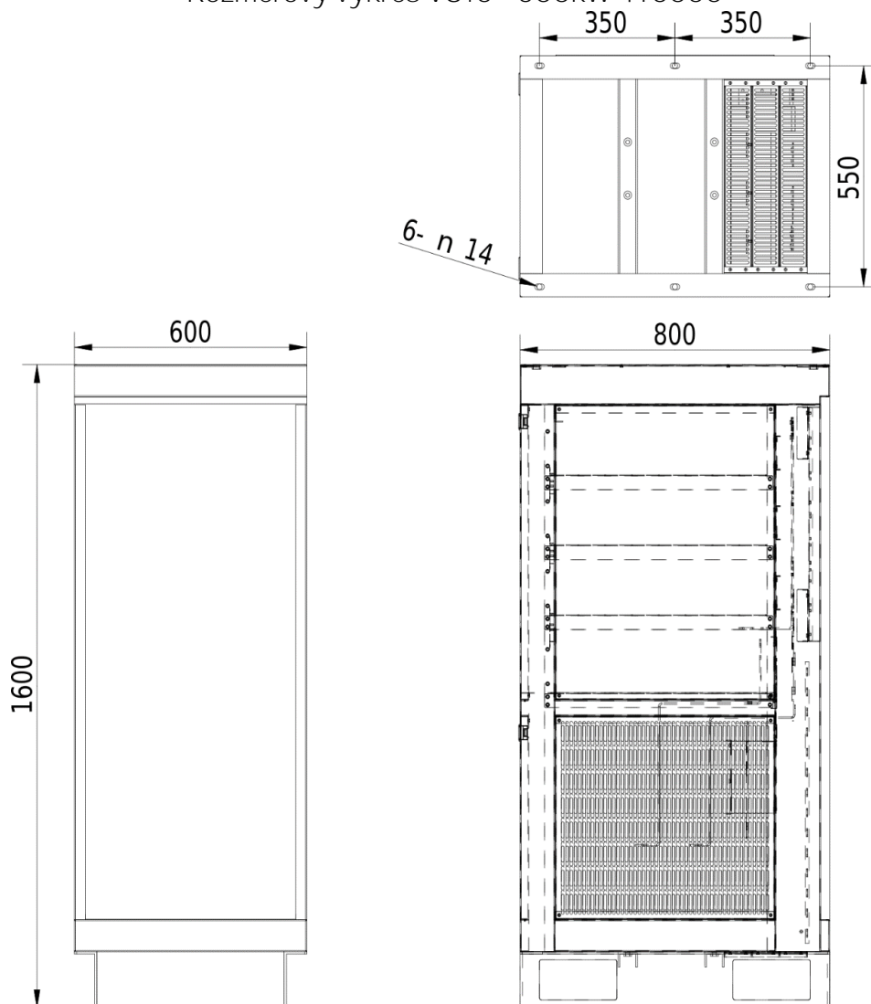
Rozmerový výkres V810 - 500kW 4T5000
