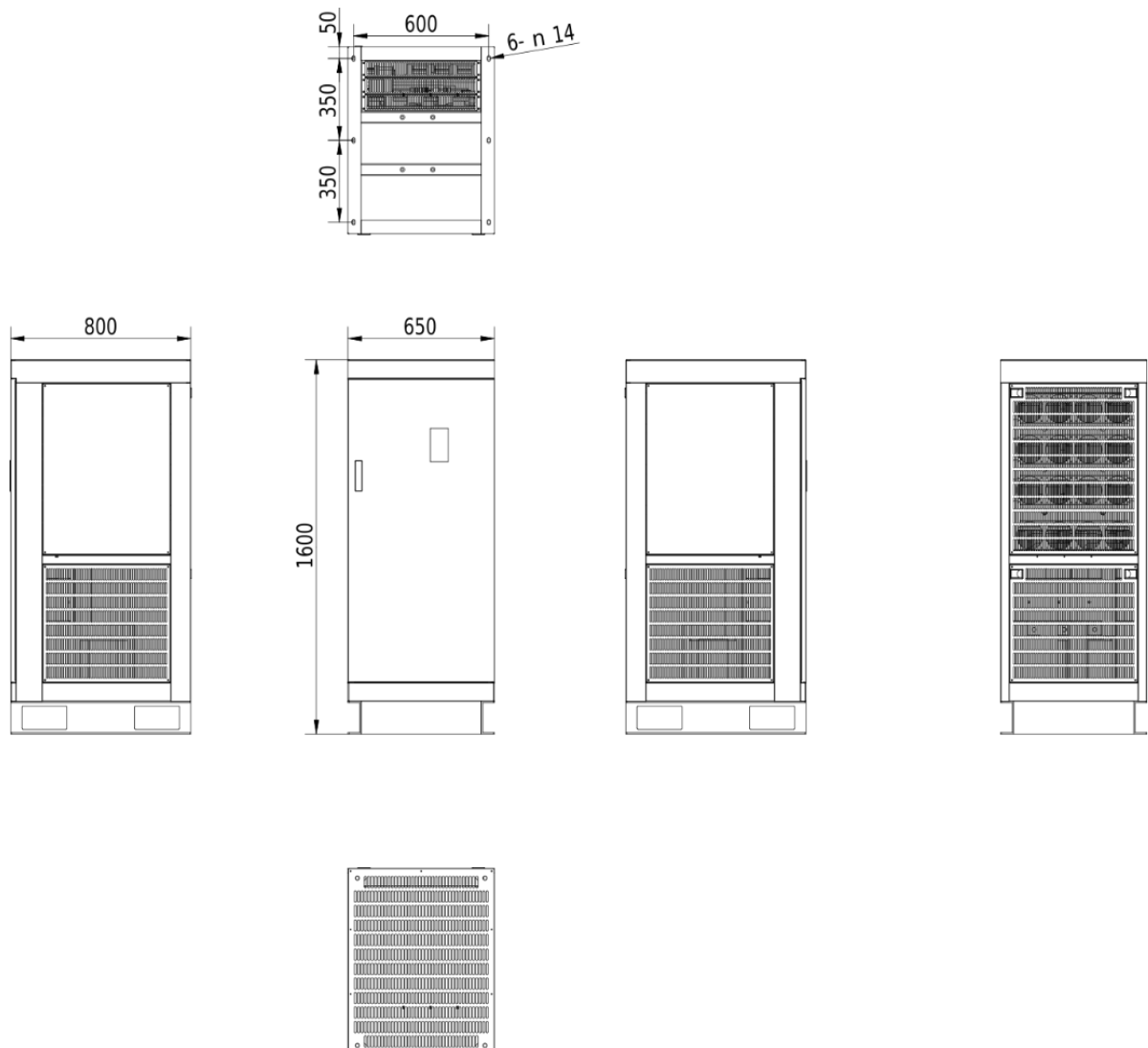
Rozmerový výkres V810 - 560kW 4T5600
