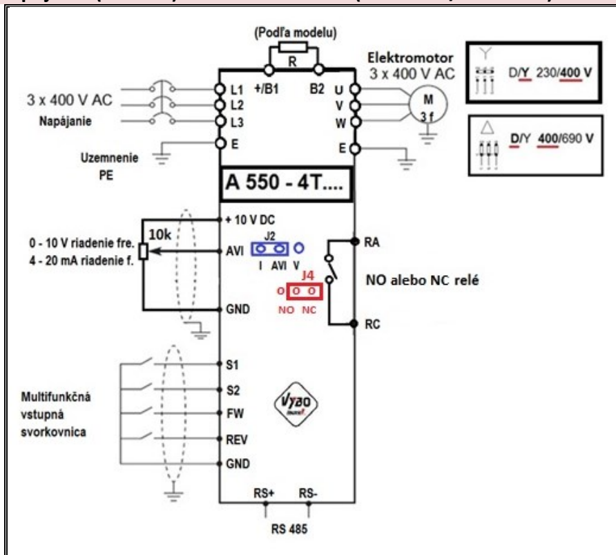
Ovládací terminál A550-4T....PLUS
