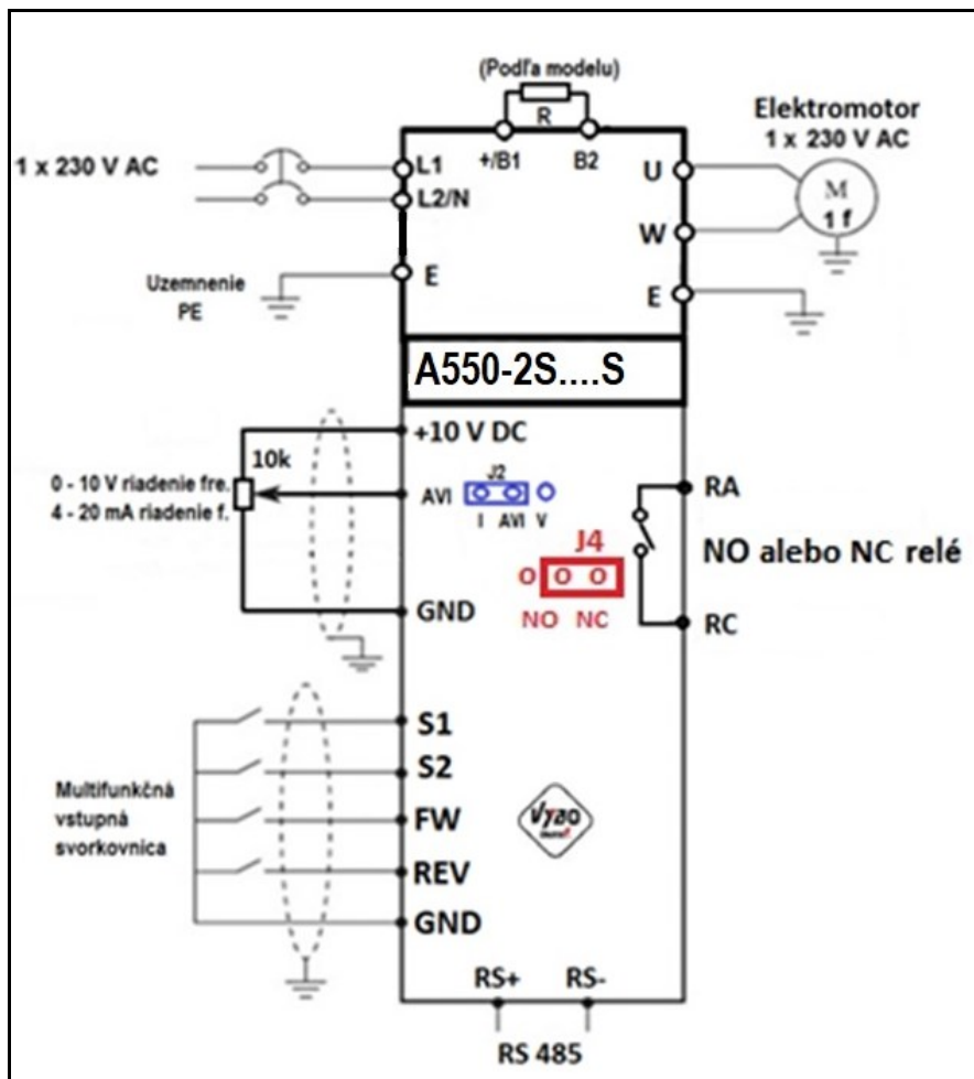
Ovládací terminál modelu A550-2S....S PLUS
