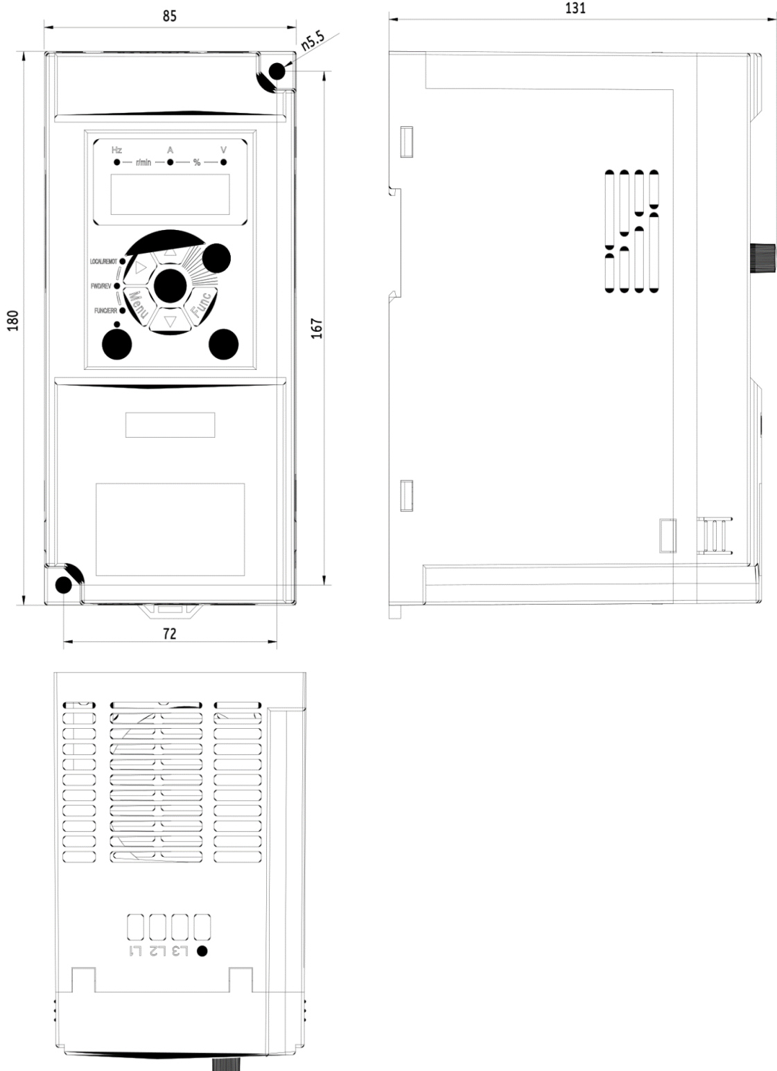
Rozmerový výkres V900 - 3,0kW 2S0030
