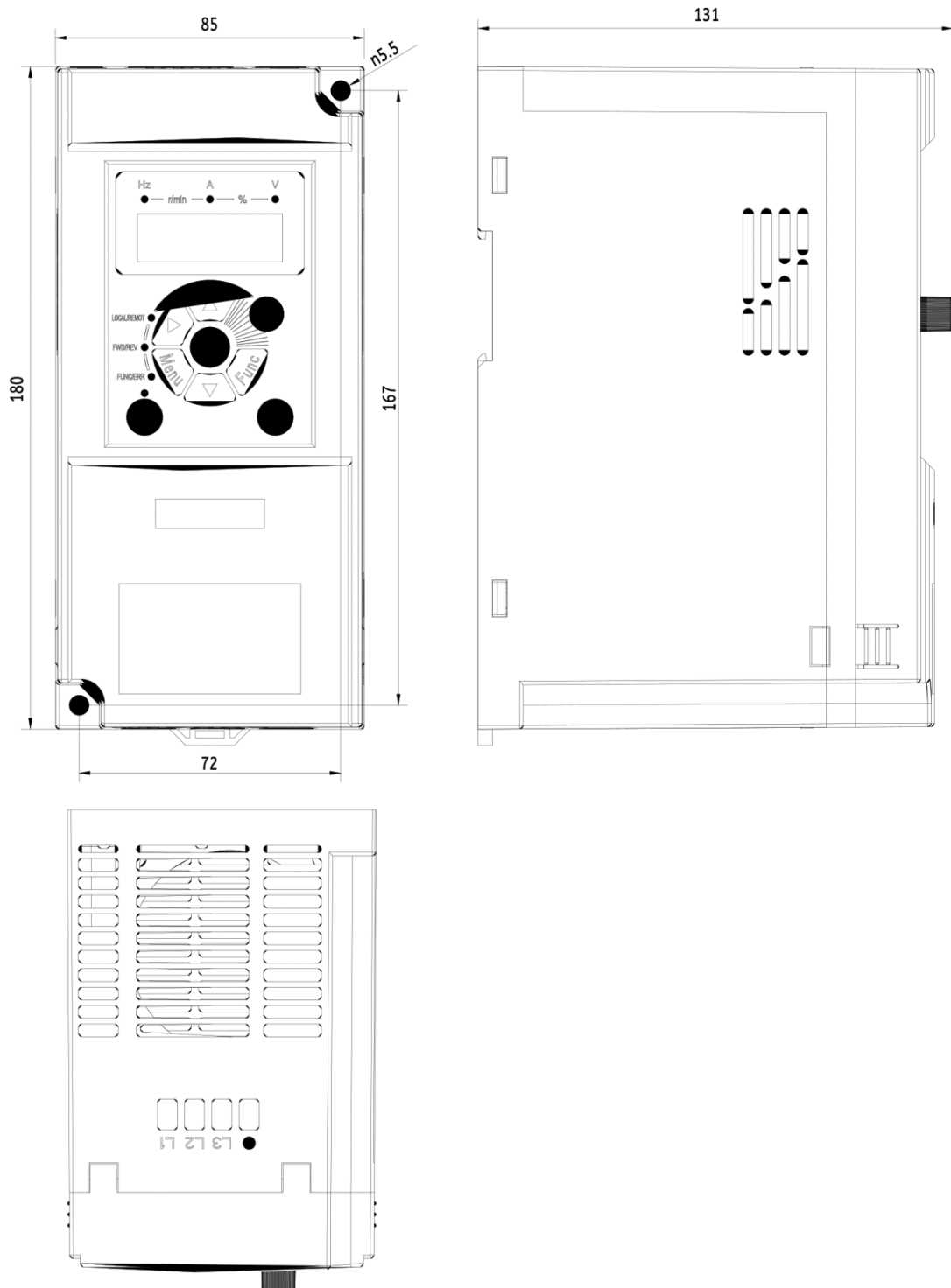
Rozmerový výkres V900 - 4,0kW 4T0040
