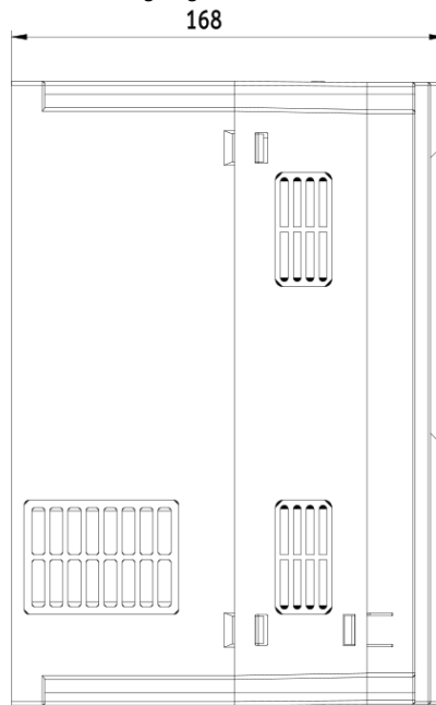
Rozmerový výkres V900 - 11kW 4T0110
