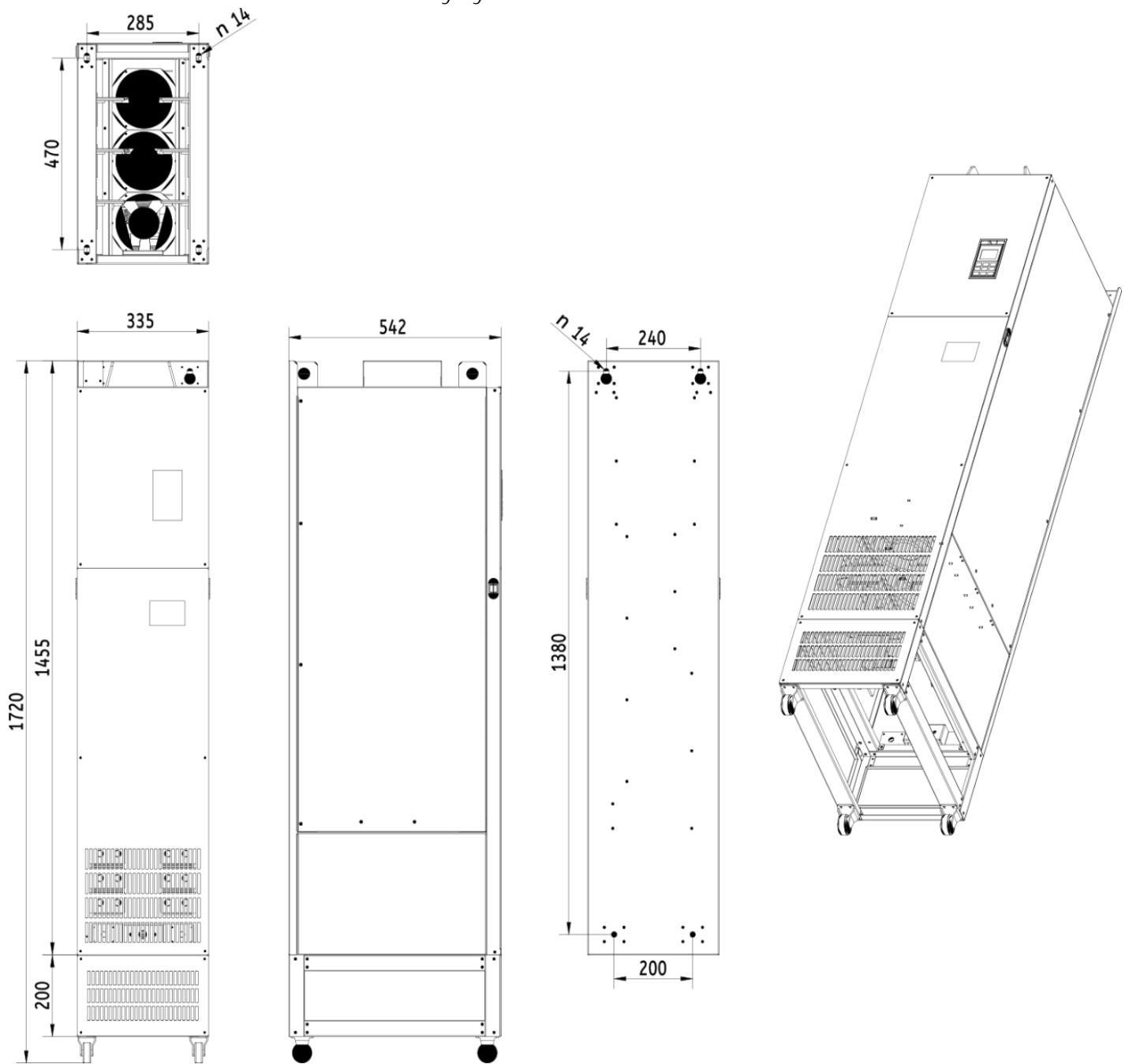
Rozmerový výkres V900 - 500kW 4T5000
