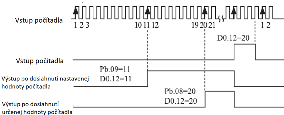
Obrázok 4-27: Dosiadnutá nastavená hodnotu počítadla
