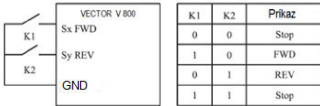
Obrázok 4-8: Nastavenie dvojvodičového režimu 1
