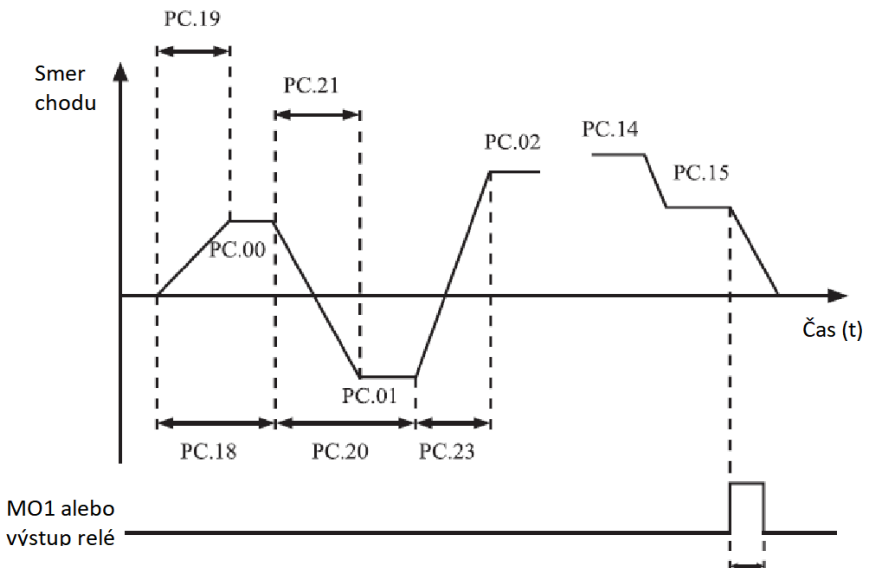
Obrázok 4-28 Jednoduchý PLC pri použití ako zdroj frekvencie
