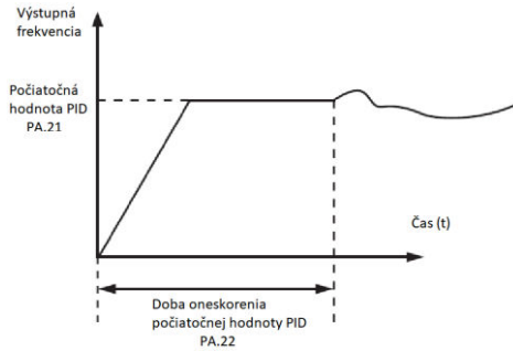
Obrázok 4-25 Funkcie počiatočnej hodnoty PID
