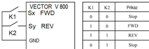
Obrázok 4-9: Nastavenie dvojvodičového režimu 1
