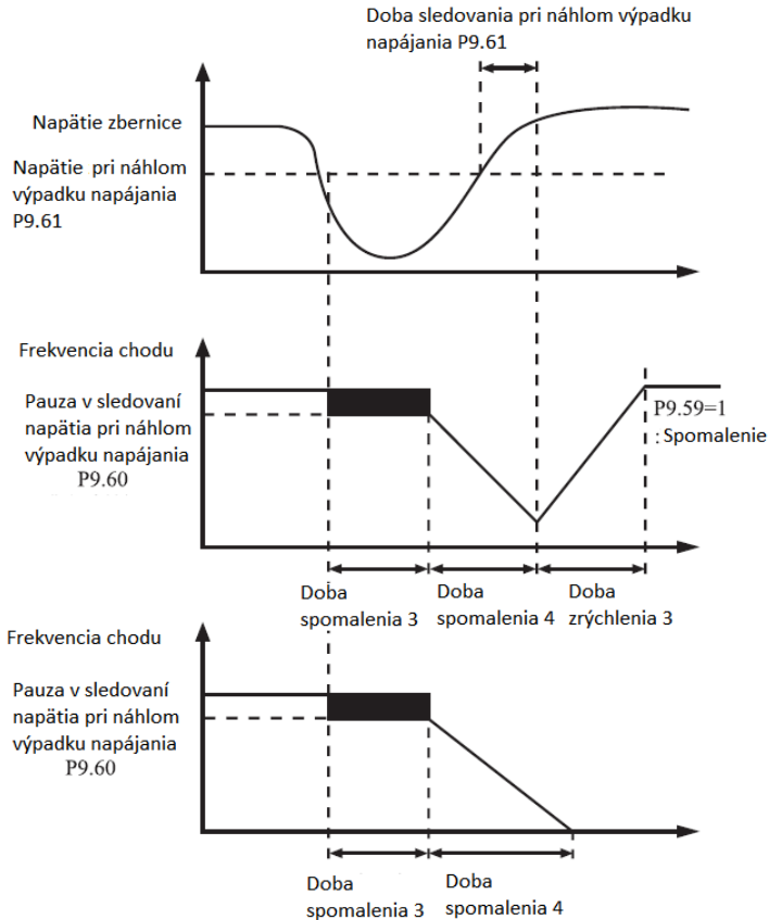
Obrázok 4-22: Činnosť meniča po náhlom výpadku napájania
