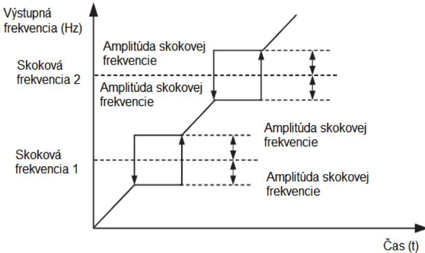
Obrázok 4-12: Princíp skokových frekvencií a amplitúdy
