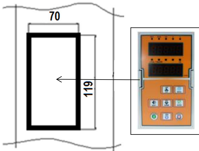
Otvor pre klávesnicu (dvojniadkový displej)
