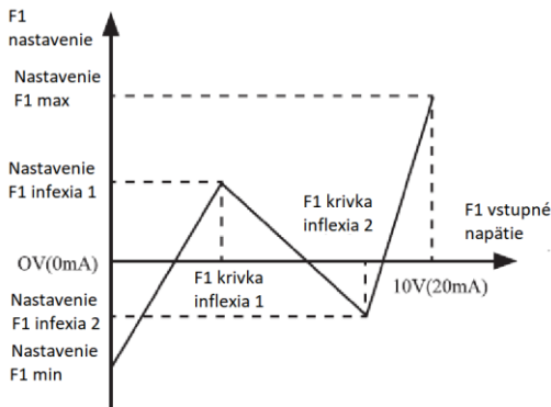
Obrázok 4-29 Schéma krivky 4 a 5
