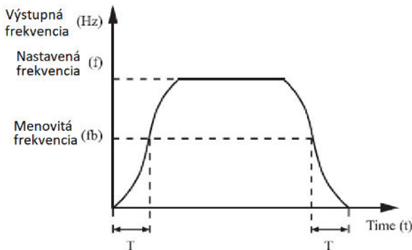
Obrázok 4-1 S-krivka zrýchlenia/spomalenia B
