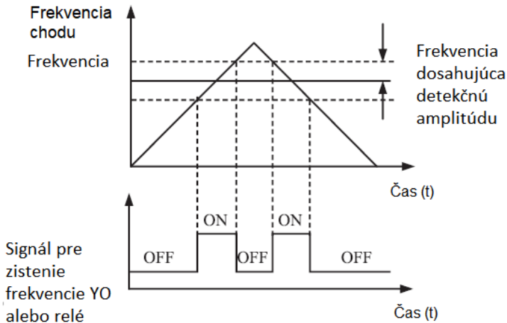
Obrázok 4-18: Detekcia akejkoľvek frekvencie
