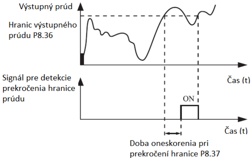
Obrázok 4-20 Detekcia prúdu
