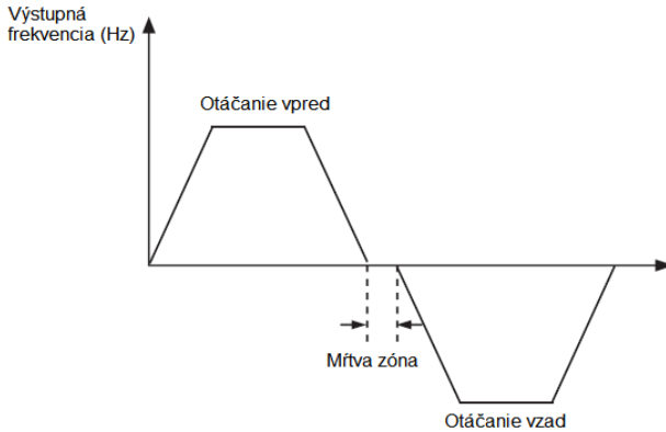
Obrázok 4-13: Otáčanie vpred / vzad
