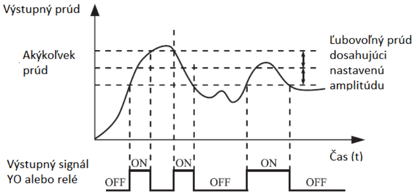
Obrázok 4-21 Detekovanie ľubovoľného prúdu
