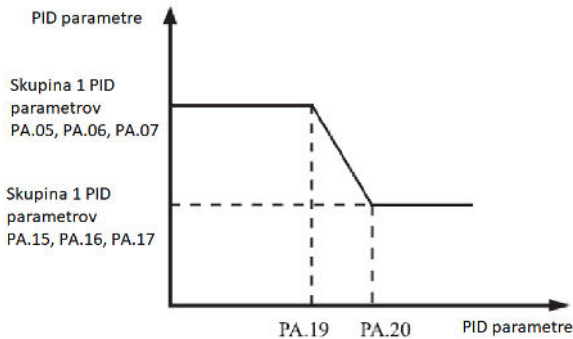
Obrázok 4-24 Prepínanie PID parametrov
