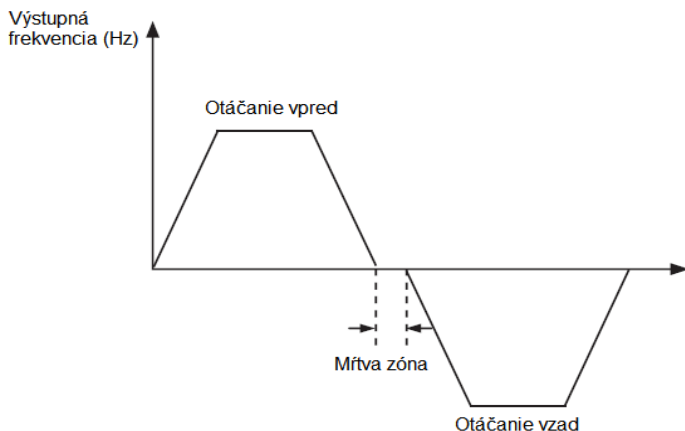
Obrázok 4-13: Otáčanie vpred / vzad
