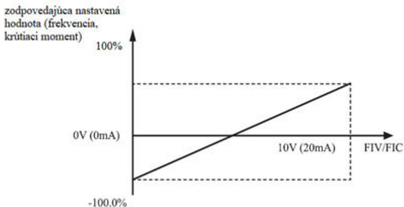
Obrázok 4-11: Vzťah medzi analógovými vstupmi a nastavenými hodnotami
