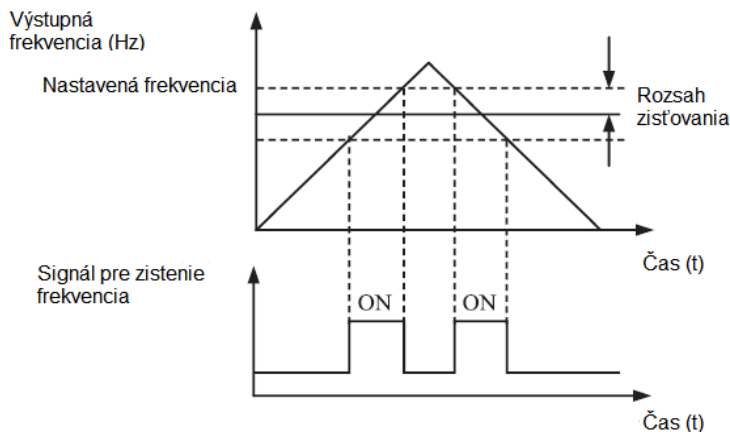
Obrázok 4-15 Rozsah detekcie frekvencie
