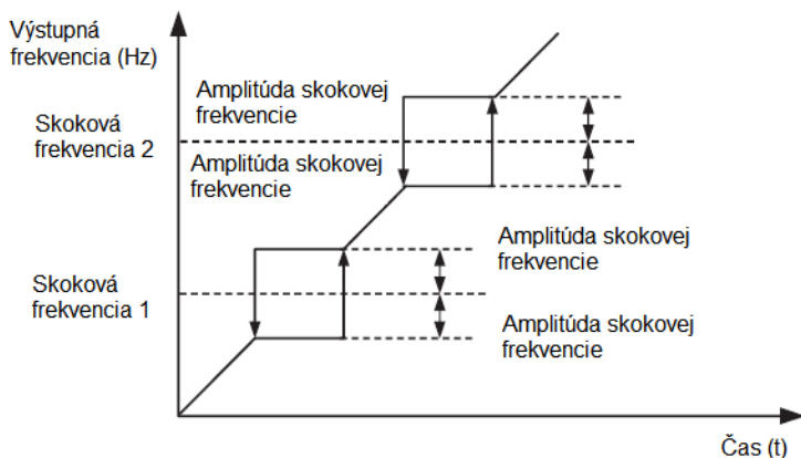
Obrázok 4-12: Princíp skokových frekvencií a amplitúdy
