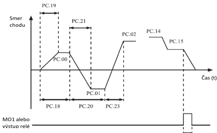
Obrázok 4-28 Jednoduchý PLC pri použití ako zdroj frekvencie
