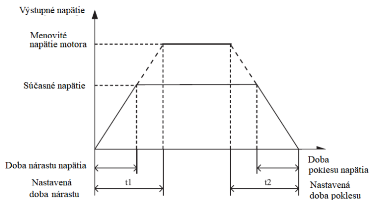
7: Pribeh napätia pri V/F separácii
